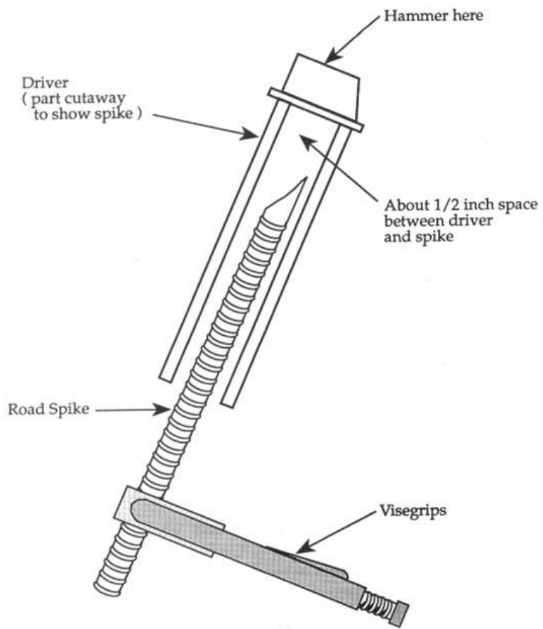
打入器（露出路钉的局部剖面图）；在这里锤击；打入器和路钉之间约 1/2 英寸的空隙；路钉；大力钳
