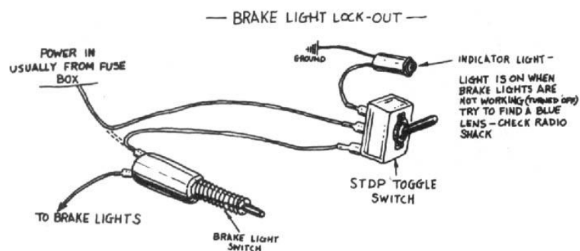
制动灯关闭器 一般来自保险丝盒的输入电源 接地
