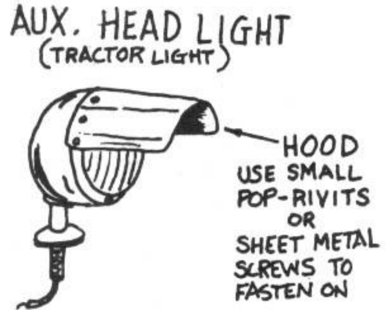
辅助前灯（拖拉机灯） 遮罩
