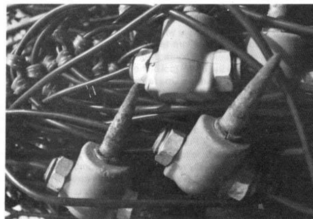
Geophones.
