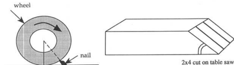
轮子；饰面钉；台锯上切割的 2x4（英寸 x 英寸）标准木料
